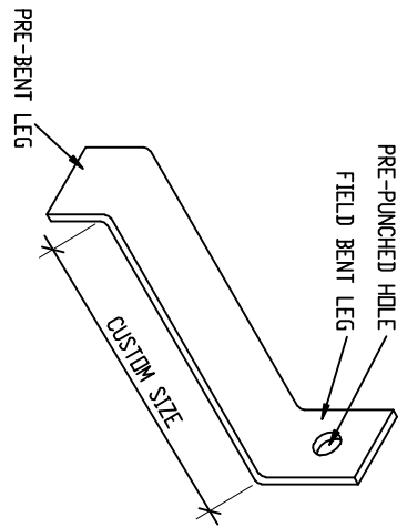
L-ANCHOR
