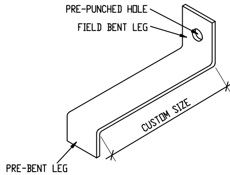
L-ANCHOR
